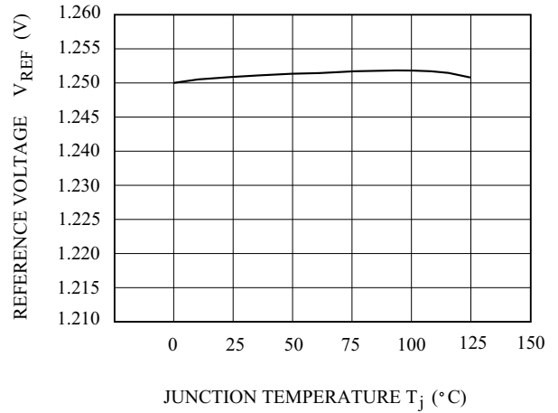
Fig. 4 V_{REF} - T_j
