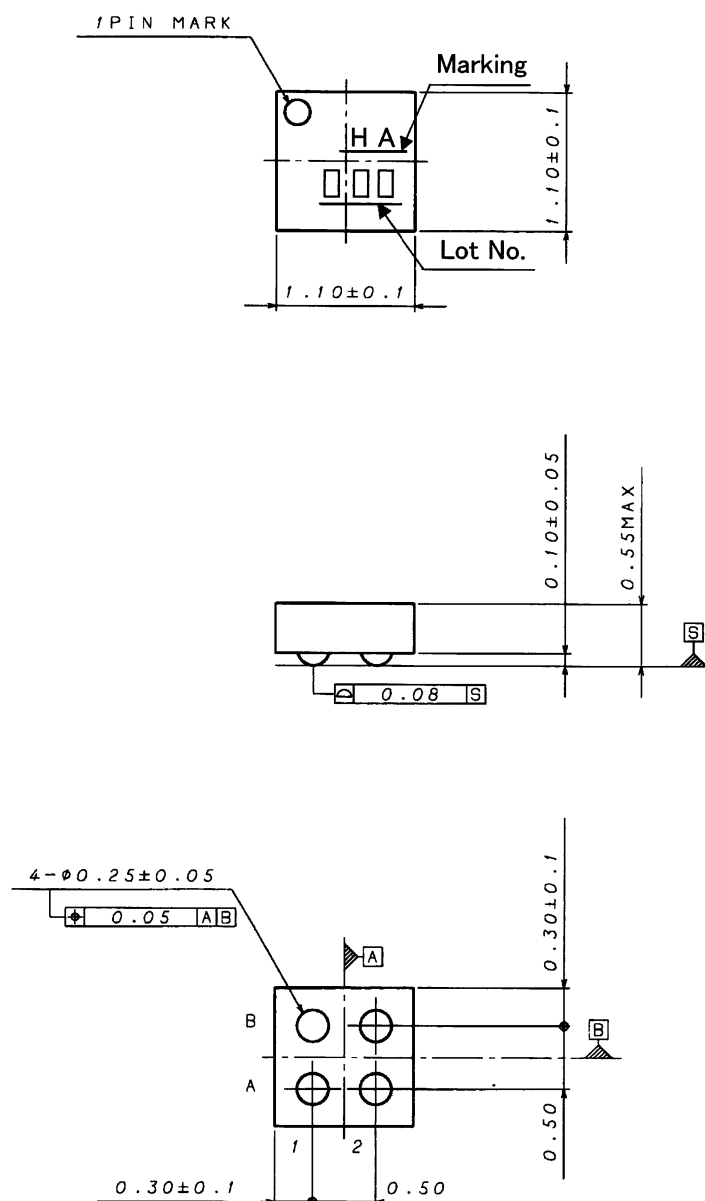
VCSP50L1 (UNIT:mm)
