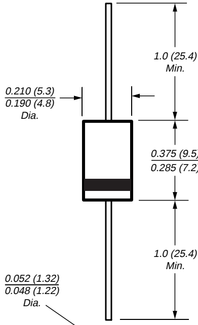
DO-201AD
