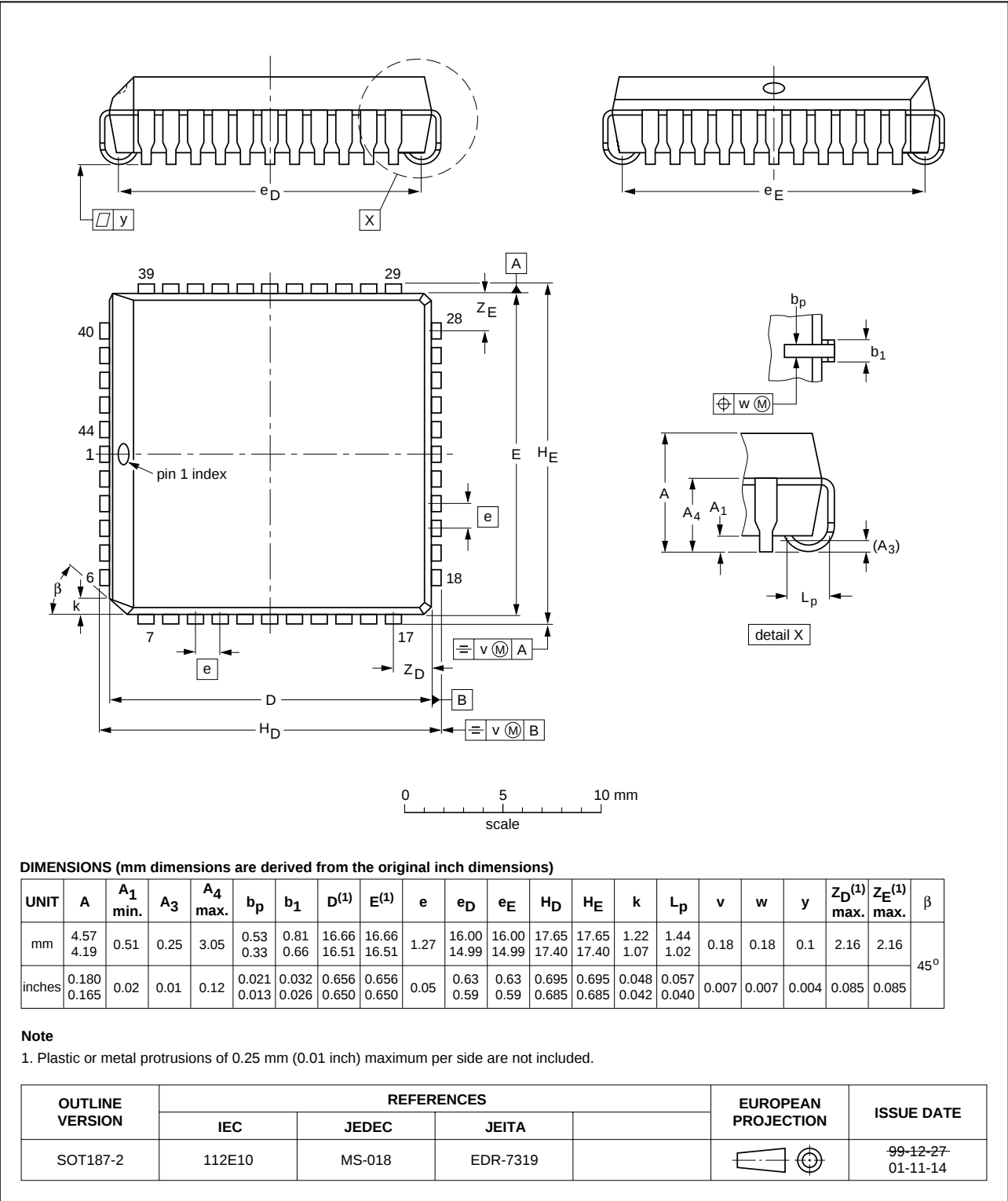
Fig 22. PLCC44 (SOT187-2).
