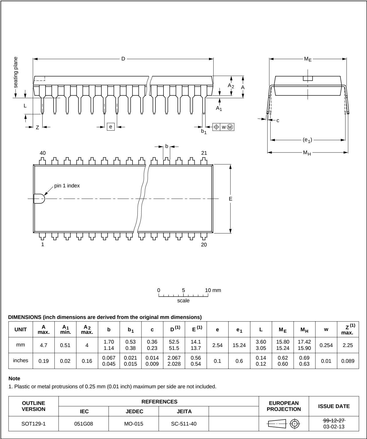
Fig 24. DIP40 (SOT129-1).
