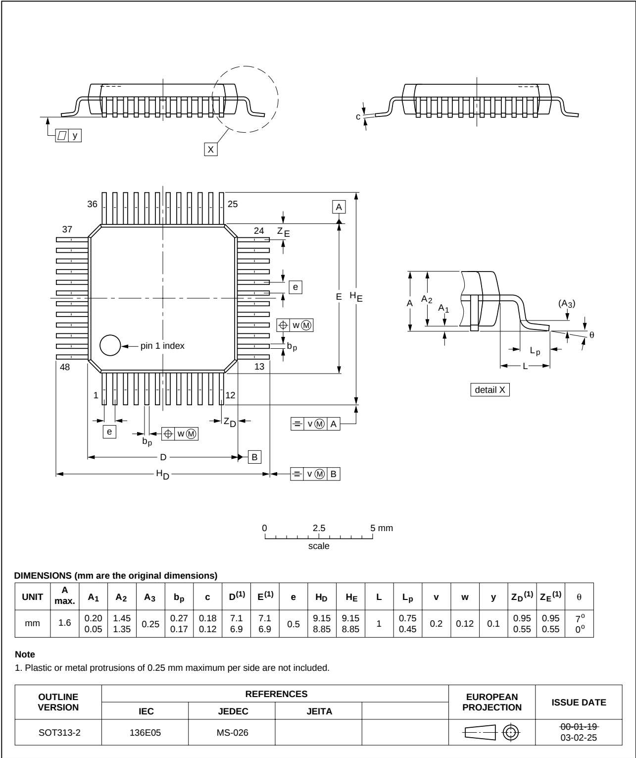
Fig 23. LQFP48 (SOT313-2).
