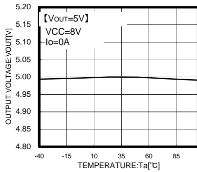
Fig. 6 Ta-VOUT
