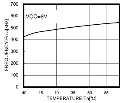
Fig.8 Ta-FOSC
