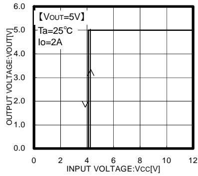
Fig.3 VCC-VOUT
