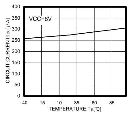
Fig.11 Ta-Icc
