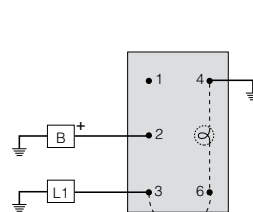
54109 dependent wiring
