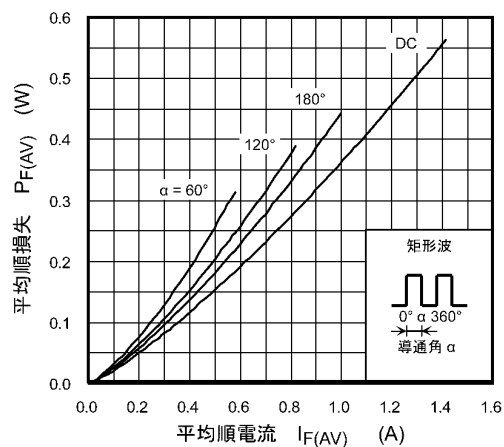
図 10.2 P_{F(AV)} - I_{F(AV)}
