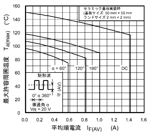
図 10.3 T_{a(max)} - I_{F(AV)}
