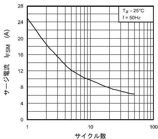
図 10.5 サージ電流
