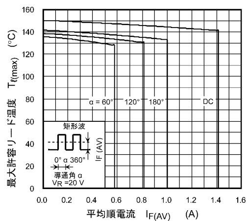
図 10.4 T_{t(max)} - I_{F(AV)}
