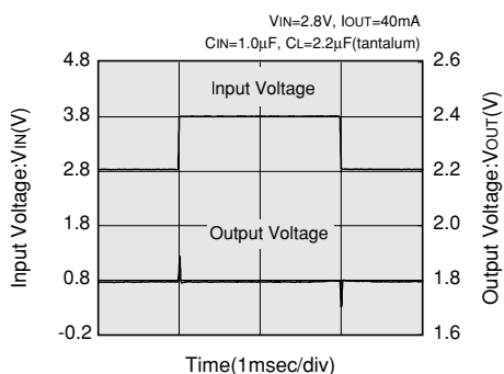
XC6201P182
