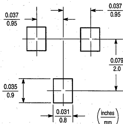
SOT-23
