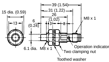
Fig. 21: E2E-X2ME□-M3/F□-M3-N
