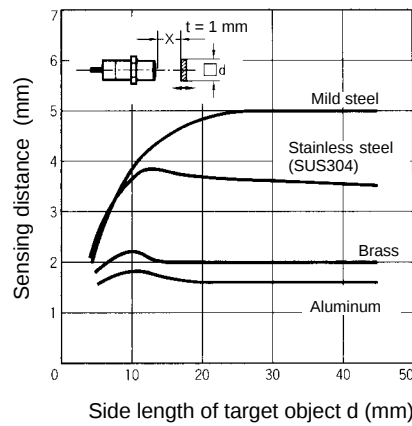
E2E-X5ME□/F□-N
