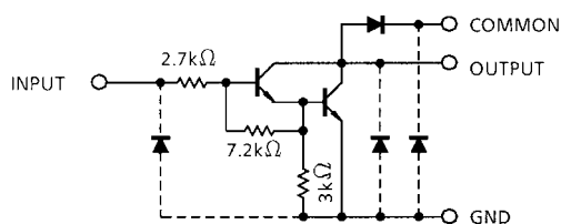
TD62003PA / APA
