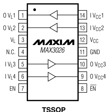
TSSOP
