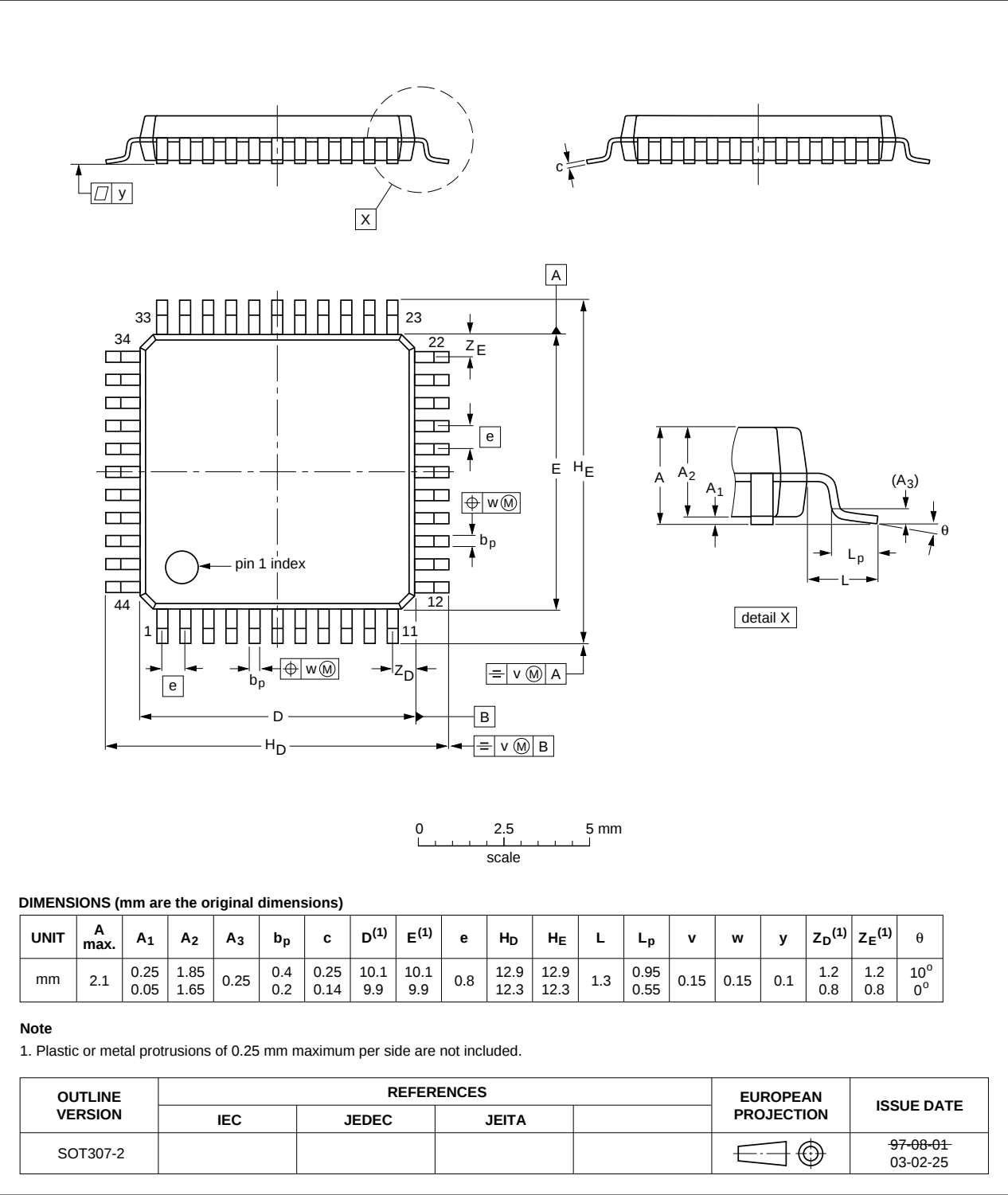
Fig 28. SOT307-2 (QFP44)
