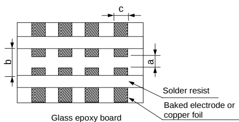
Fig.3 (in:mm)
