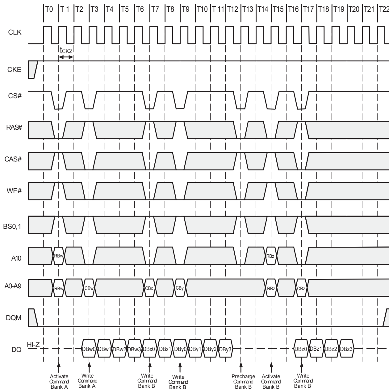
(Burst Length=4,CAS#Latency=2)
