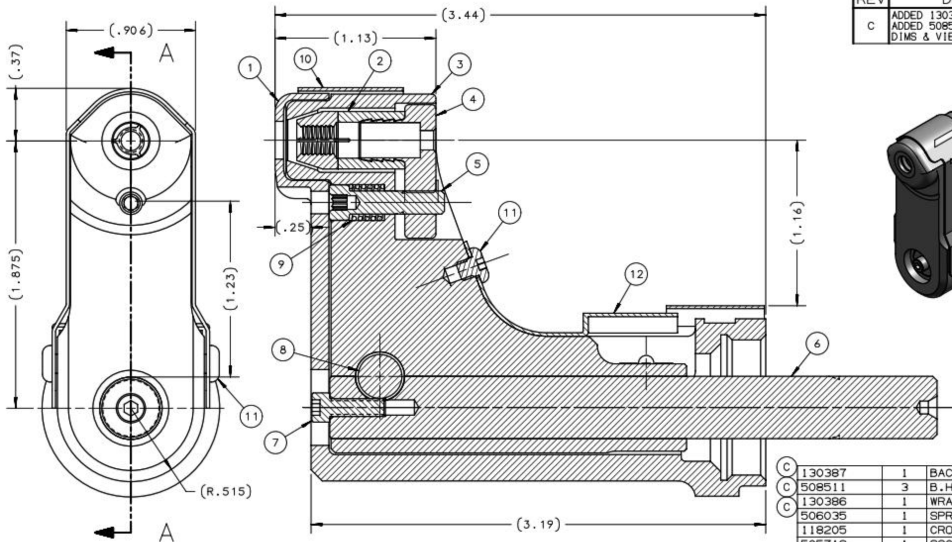
SECTION A-A
