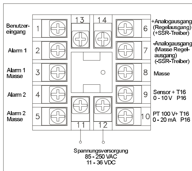
Rückseite T16/P16
