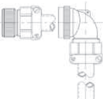
CIR06...straight CIR08...90°
