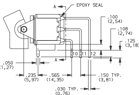
.190 TYP. (4, 83) .050 TYP. (1, 27) TERM. WIDTH Actuator Shown In Pos. 1
