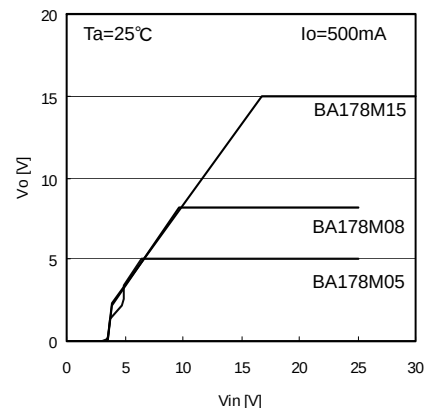
Fig.3 電源電圧－出力電圧 (Io=500mA)
