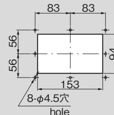
パネル穴明け寸法 (1/2) Panel drilling dimension
