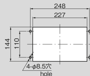
パネル穴明け寸法 (1/2) Panel drilling dimension
