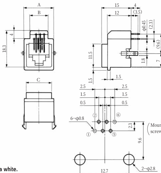
TM3RA-6*(50)
