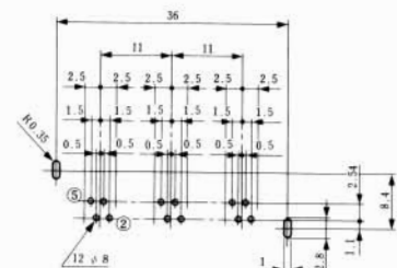
TM2RE-1812(50)
