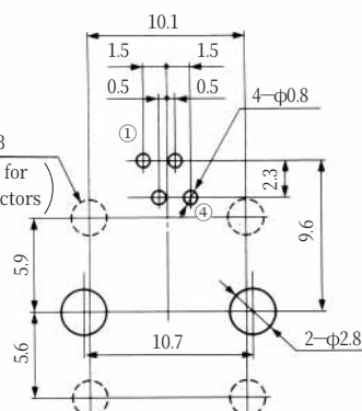
TM3RA-44
