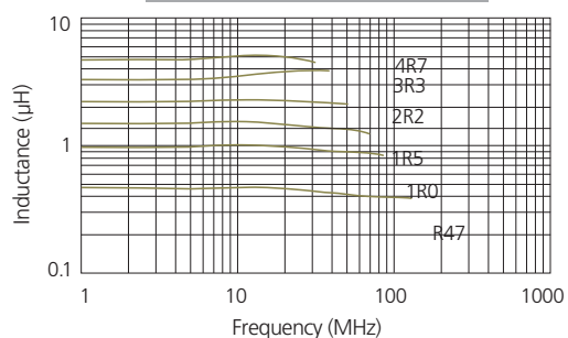
INDUCTANCE(Typ.)
