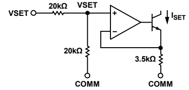
Figure 29. VSET Interface
