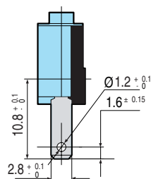
W7A5 / W7S
