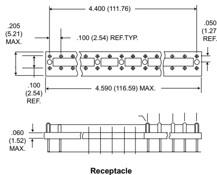
Receptacle
