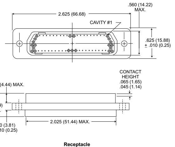
Receptacle
