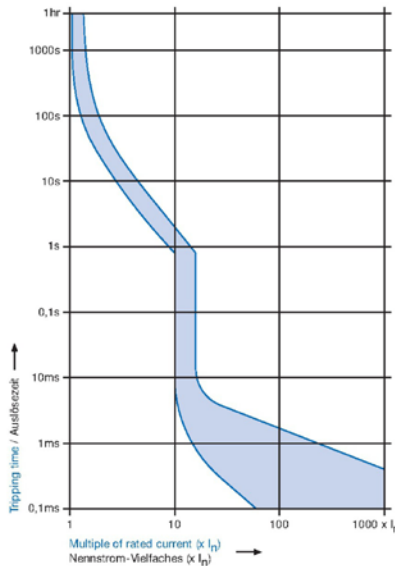
Tripping characteristic DG Auslösekennlinie DG
