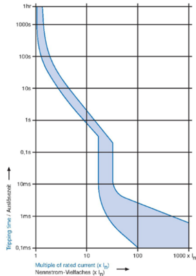
Tripping characteristic DH Auslösekennlinie DH
