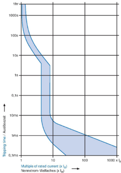
Tripping characteristic DF Auslösekennlinie DF
