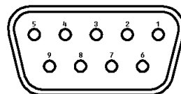
Sub-D 9 pin
