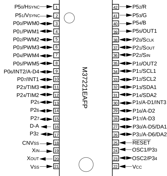
Outline 42P2R-A/E
