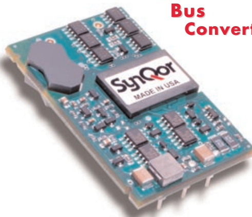
BQ50120QTA25 Module
