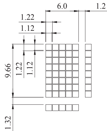
DOT SIZE
