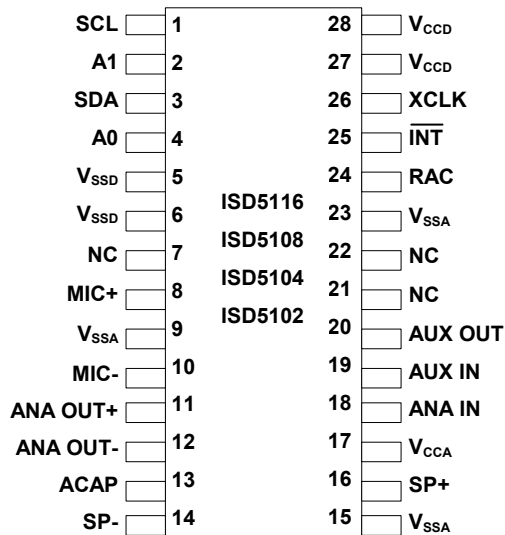
SOIC
