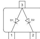
BAS40-06 BAS40-06W
