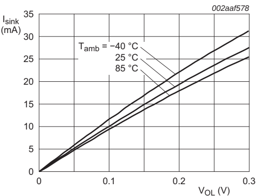
a. V_{\text{DD(P)}} = 1.65\text{ V}
