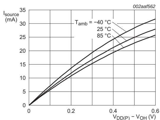
b. V_{\text{DD(P)}} = 1.8\text{ V}
