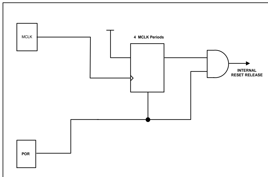
Figure 4 POR Circuit
