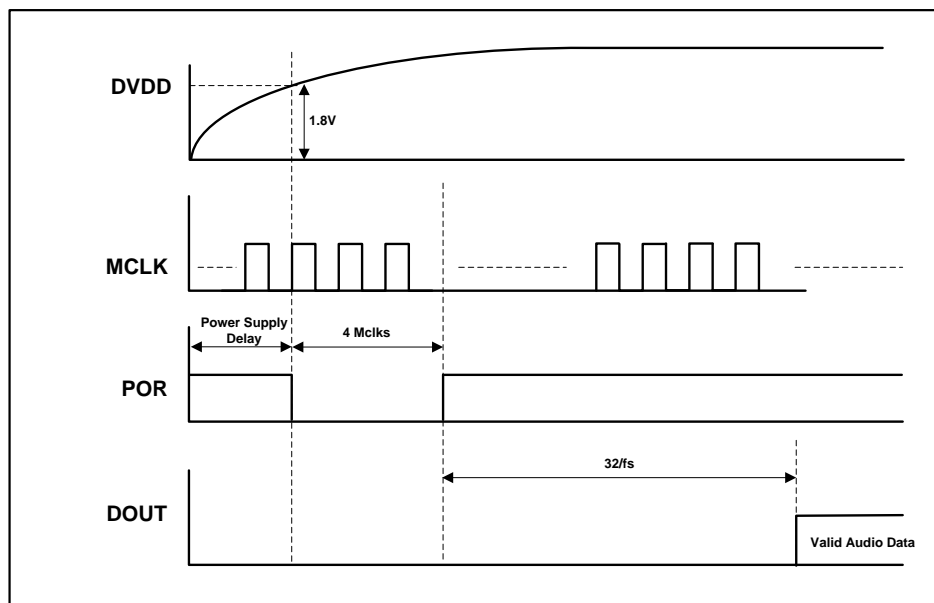
Figure 5 POR Timing
