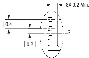
Detail D Scale: 1X
