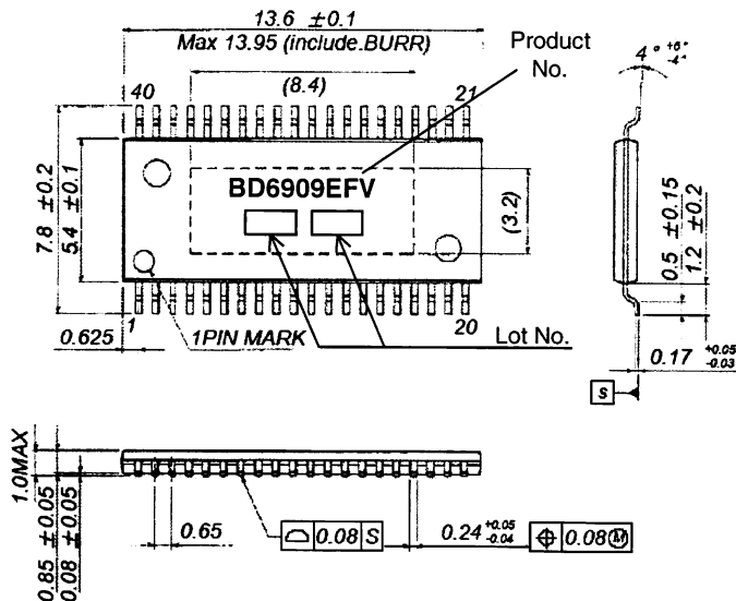
HTSSOP-B40 (Unit:mm)
