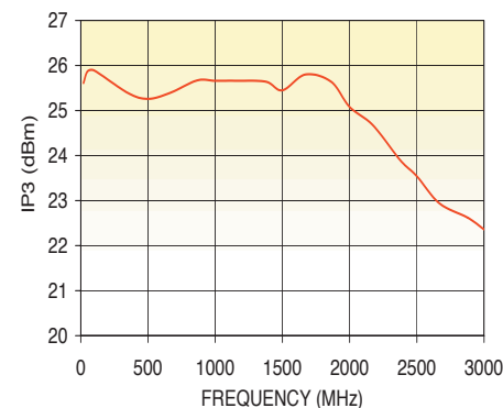
ZX60-3018G IP3
