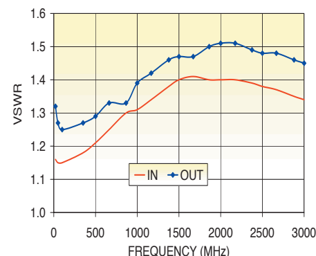
ZX60-3018G VSWR
