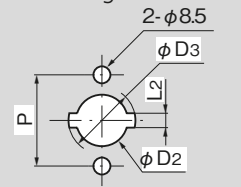
パネル穴明け寸法 Panel drilling dimensions
