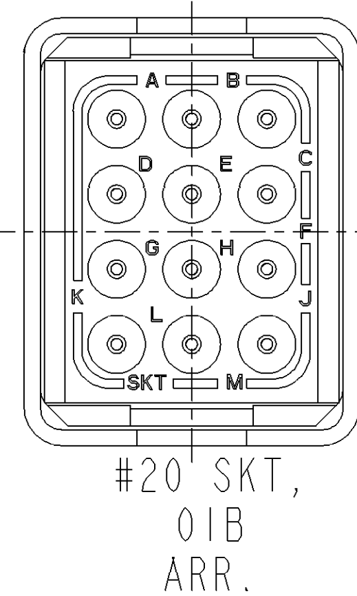
GROMMET VIEWS
