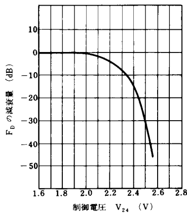
F_D - V_{24} (フェード特性)
