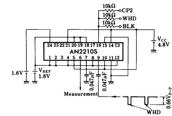
Test Circuit 7 (V O(EXT.Nega.) )
