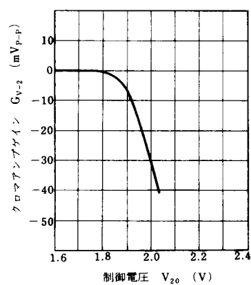
G_V - V_{20} (クロマゲインコントロール)
