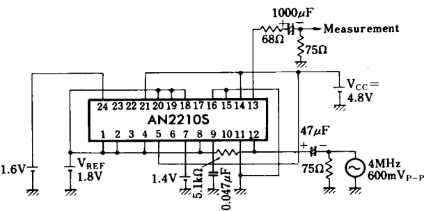
Test Circuit 11 (v O(Sync.) )
