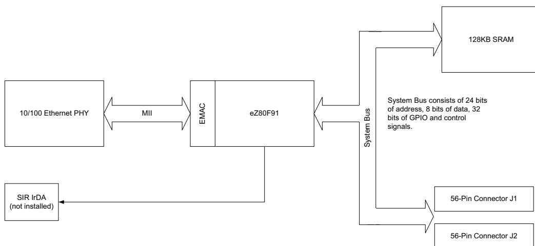
Figure 1. eZ80F91 Mini Enet Module for eZ80AcclaimPlus! Block Diagram
