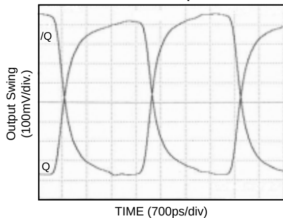
200MHz Output
