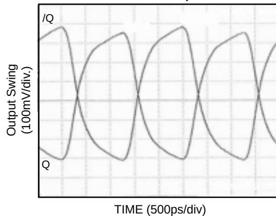
400MHz Output
