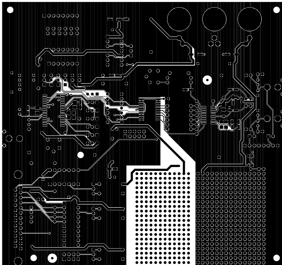
TOP SIDE
