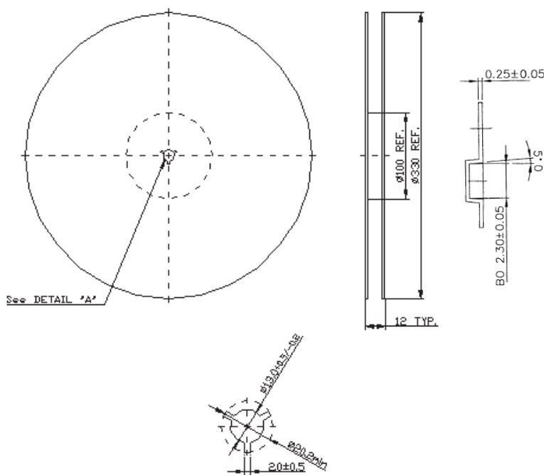
Reel Dimensions
