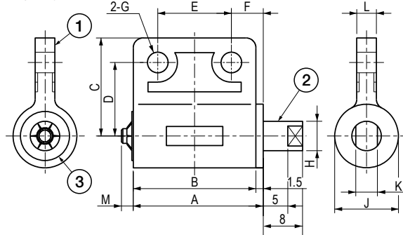
ヒンジ Hinge only
