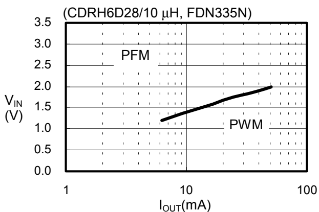
(31) S-8341C25AFT
