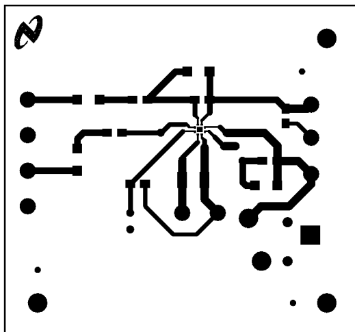
Figure 23. Bottom Layer
