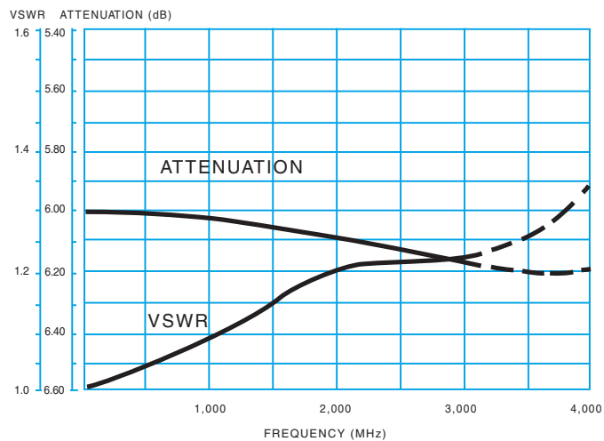
6 dB ATTENUATOR
