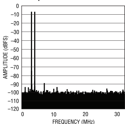
LTC2265-12: 8k Point 2-Tone FFT, f_{IN} = 68\text{MHz} , 69\text{MHz} , -1\text{dBFS} , 65\text{Mps}
