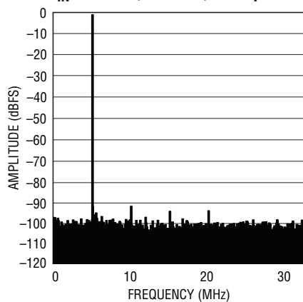
LTC2265-12: 8k Point FFT, f_{IN} = 70\text{MHz} , -1\text{dBFS} , 65\text{Mps}
