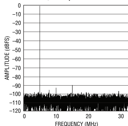
LTC2265-12: 8k Point FFT, f_{IN} = 5\text{MHz} , -1\text{dBFS} , 65\text{Mps}
