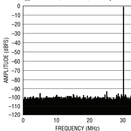
LTC2265-12: 8k Point FFT, f_{IN} = 30\text{MHz} , -1\text{dBFS} , 65\text{Mps}
