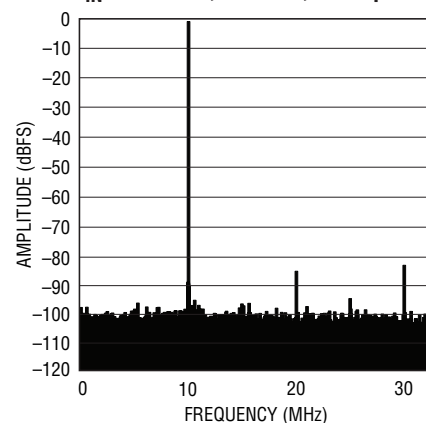
LTC2265-12: 8k Point FFT, f_{IN} = 140\text{MHz} , -1\text{dBFS} , 65\text{Mps}
